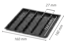
Alvéole 5 rangées 160 x 160 mm INFALV1616NO5RA
